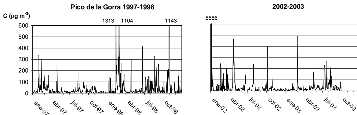
Figura 1.- Variabilidad de la carga de polvo (en µg m -3 ) durante los períodos 1997-1998 y 2002-2003 en Gran Canaria (1980 m)
