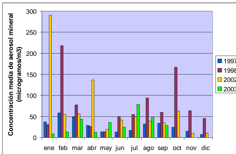
Figura 2.- Variabilidad mensual de las concentraciones de aerosol mineral ( \mu\text{g m}^{-3} ) en el aire medidas en el Pico de la Gorra
